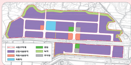
동두천 국가산업단지 토지이용계획도
